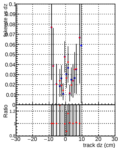
—•— DQM_mkFit_TT_base —•— DQM_mkFit_TT_retrain
