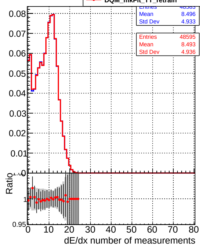
DQM_mkFit_TT_base DQM_mkFit_TT_retrain
