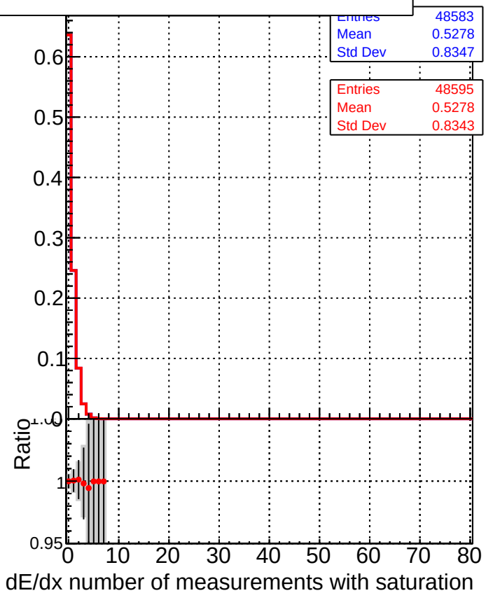
DQM_mkFit_TT_base DQM_mkFit_TT_retrain
