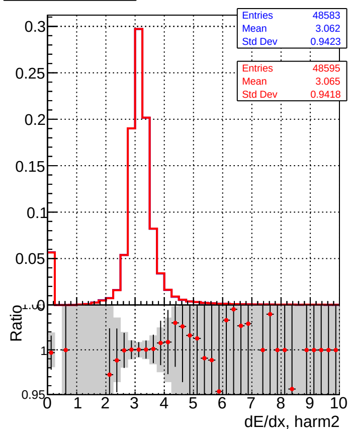
DQM_mkFit_TT_base DQM_mkFit_TT_retrain
