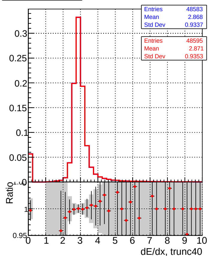
DQM_mkFit_TT_base DQM_mkFit_TT_retrain
