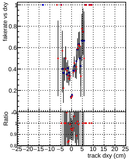
—●— DQM_mkFit_TT_base —●— DQM_mkFit_TT_retrain
