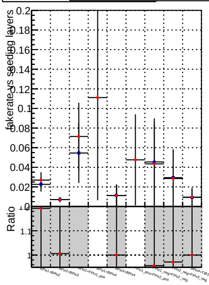
Fake rate vs. —•— DQM mkFit TT_base —•— DQM mkFit TT_retrain
