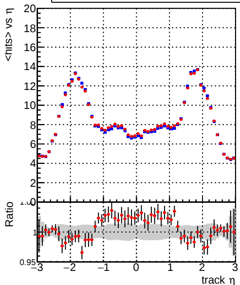
— DQM_mkFit_TT_base — DQM_mkFit_TT_retrain
