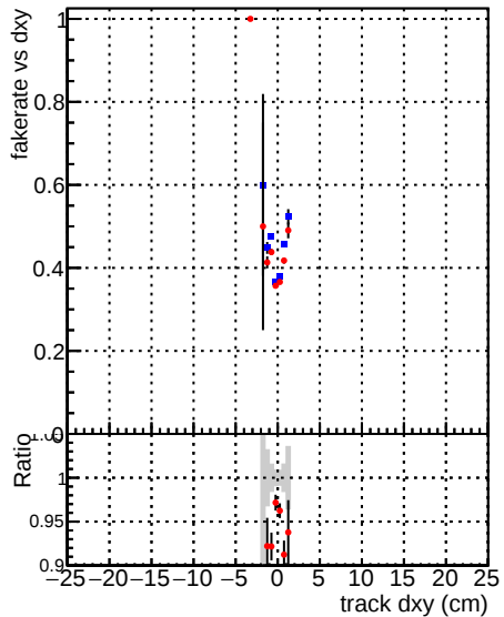
—●— DQM_mkFit_TT_base —●— DQM_mkFit_TT_retrain
