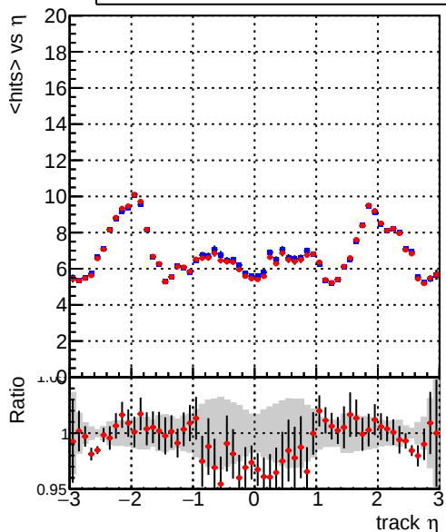
DQM_mkFit_TT_base mean hits DQM_mkFit_TT_retrain
