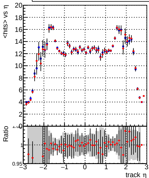
— DQM_mkFit_TT_base — DQM_mkFit_TT_retrain mean hits
