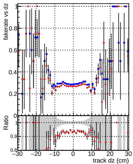
—●— DQM_mkFit_TT_base —●— DQM_mkFit_TT_retrain
