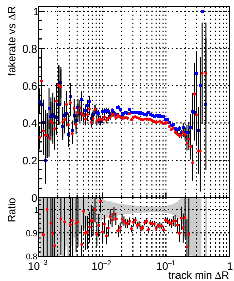
—●— DQM_mkFit_TT_base —●— DQM_mkFit_TT_retrain
