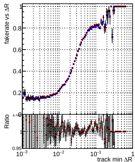
Legend: DQM mkFit TT base DQM mkFit TT retrain DQM mkFit TT retrain_noCandDNN
