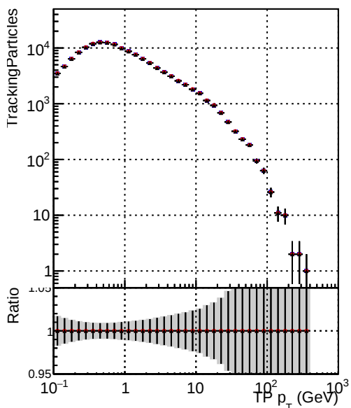
—•— DQM_mkFit_TT_base —•— DQM_mkFit_TT_retrain —•— DQM_mkFit_TT_retrain_noCandDNN
