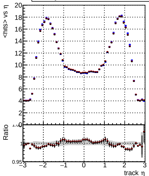
— DQM_mkFit_TT_base — DQM_mkFit_TT_retrain — DQM_mkFit_TT_retrain_noCandDNN mean hits
