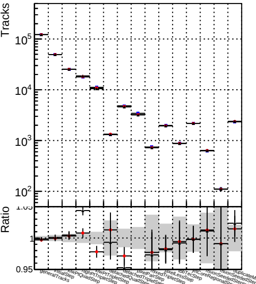
Legend: ■ DQM_mkFit_TT_base ● DQM_mkFit_TT_retrain ■ DQM_mkFit_TT_retrain_noCandDNN
