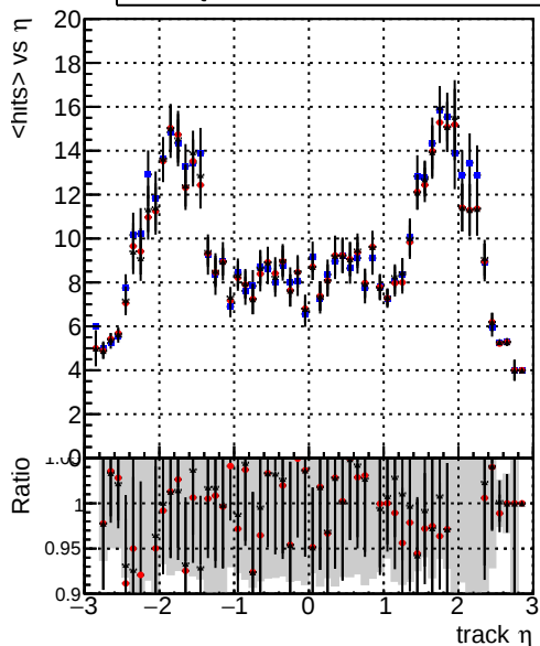
mean hits — DQM_mkFit_TT_base — DQM_mkFit_TT_retrain — DQM_mkFit_TT_retrain_noCandDNN
