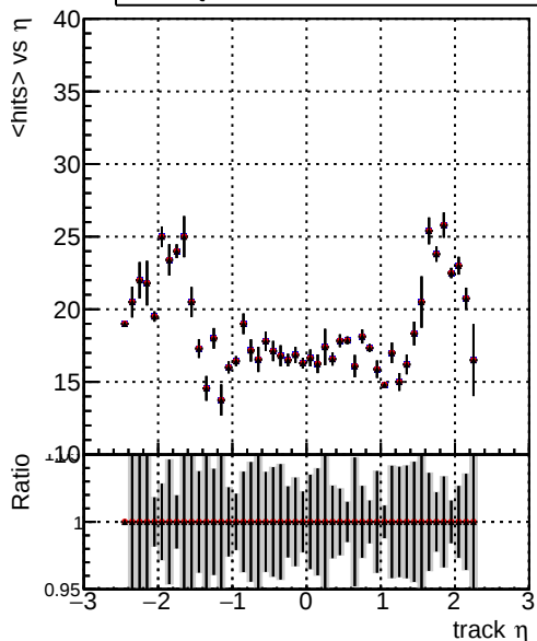
DQM_mkFit_TT_base DQM_mkFit_TT_retrain DQM_mkFit_TT_retrain_noCandDNN mean hits
