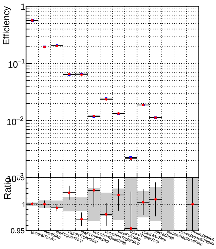
DQM_CKF_TT_base DQM_CKF_TT_retrain
