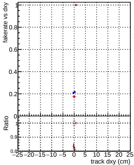
—●— DQM_CKF_TT_base —●— DQM_CKF_TT_retrain
