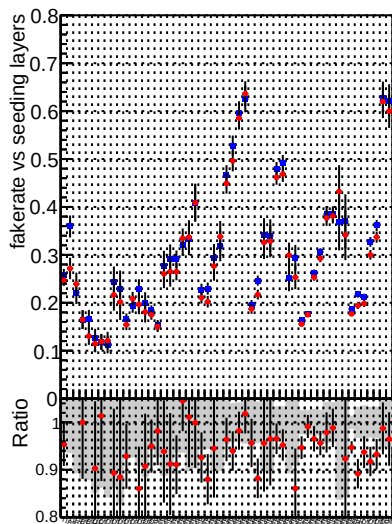
Fake rate vs. —♦— DQM CKF TT_base —★— DQM CKF TT_retrain
