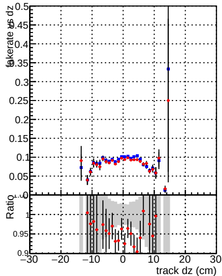
Fake rate vs dz —●— DQM CKF TT_base —●— DQM CKF TT_retrain
