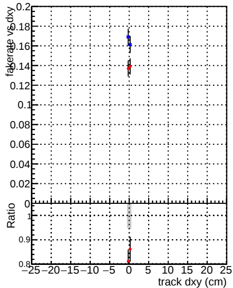
—●— DQM_CKF_TT_base —●— DQM_CKF_TT_retrain
