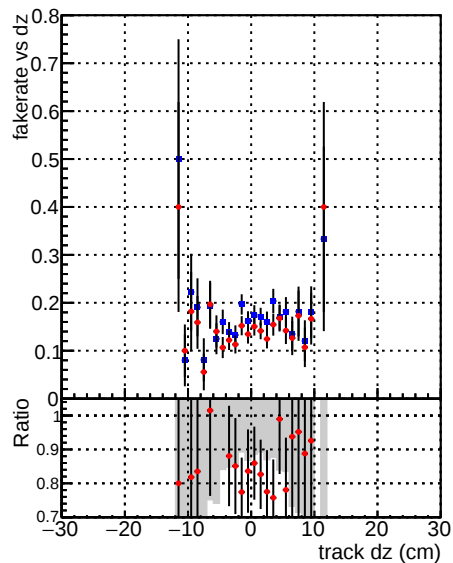
—●— DQM_CKF_TT_base —●— DQM_CKF_TT_retrain
