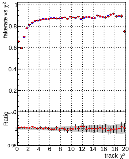
Fake rate vs. —•— DQM CKF TT_base —•— DQM CKF TT_retrain
