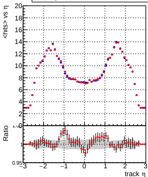
mean hits DQM_CKF_TT_base DQM_CKF_TT_retrain
