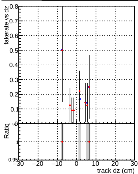
—●— DQM_CKF_TT_base —●— DQM_CKF_TT_retrain
