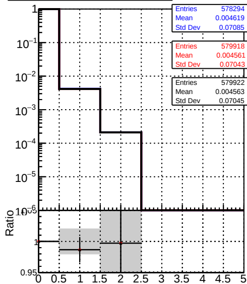
mean hits — DQM_mkFit_TT_base — DQM_mkFit_TT_retrain_noCandDNN — DQM_mkFit_TT_retrain
