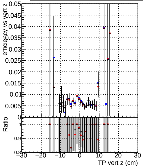
Efficiency vs vert z —●— DQM_mkFit_TT_base —●— DQM_mkFit_TT_retrain_noCandDNN —●— DQM_mkFit_TT_retrain
