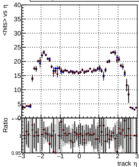
mean hits — DQM_mkFit_TT_base — DQM_mkFit_TT_retrain_noCandDNN — DQM_mkFit_TT_retrain
