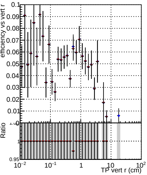
Efficiency vs TP vert r (cm) DQM_mkFit_TT_base DQM_mkFit_TT_retrain_noCandDNN DQM_mkFit_TT_retrain
