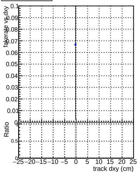
—•— DQM CKF QCDHighPt_retrain —•— DQM mkFit QCDHighPt_retrain
