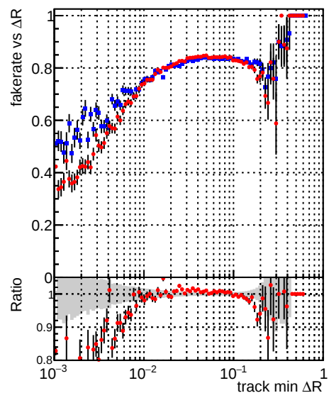
■ DQM_CKF_QCDHighPt_retrain ■ DQM_mkFit_QCDHighPt_retrain
