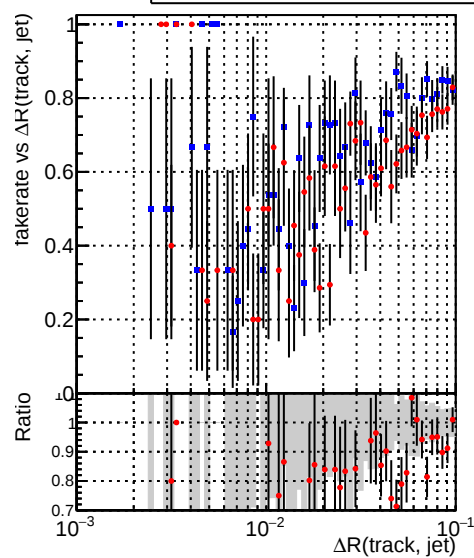
■ DQM_CKF_QCDHighPt_retrain ■ DQM_mkFit_QCDHighPt_retrain
