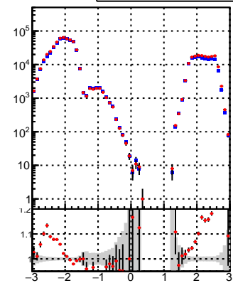
—●— DQM_mkFit —+— DQM_BDT_mkFit
