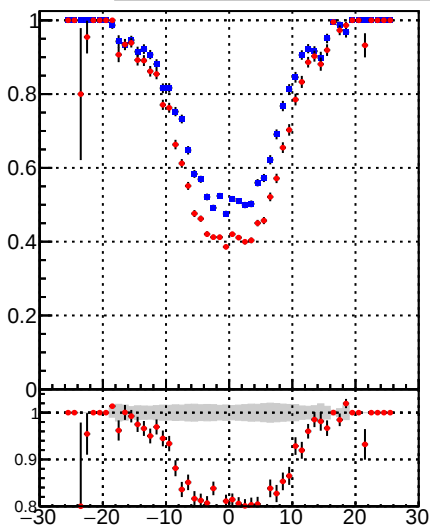
—•— DQM_mkFit —+— DQM_BDT_mkFit
