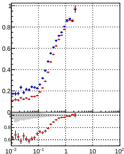
—•— DQM_mkFit —+— DQM_BDT_mkFit
