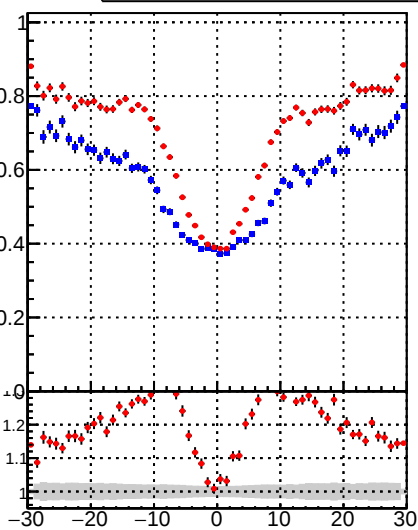
■ DQM_mkFit ● DQM_BDT_mkFit
