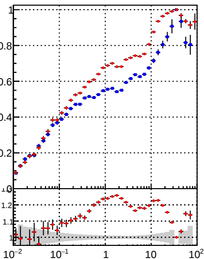
■ DQM_mkFit ● DQM_BDT_mkFit
