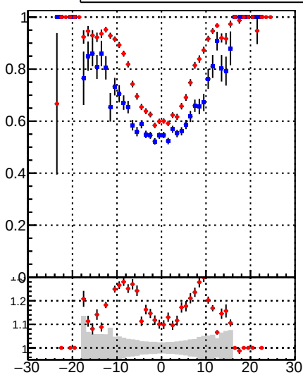
—●— DQM_mkFit —×— DQM_BDT_mkFit
