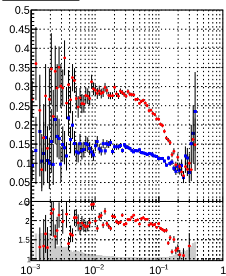
— DQM_mkFit — DQM_BDT_mkFit
