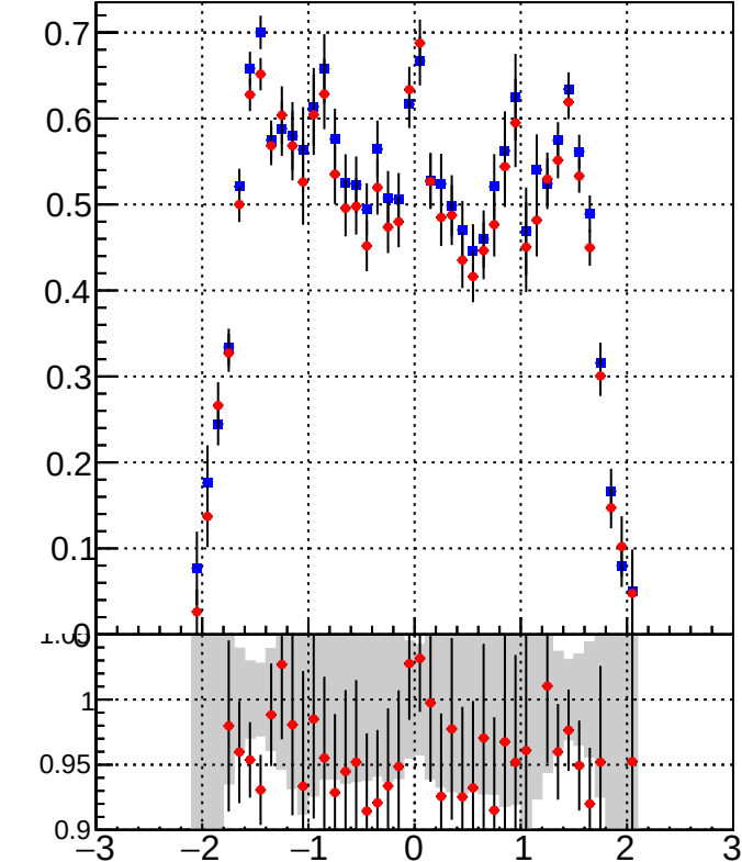
mean # PXL hits vs eta
