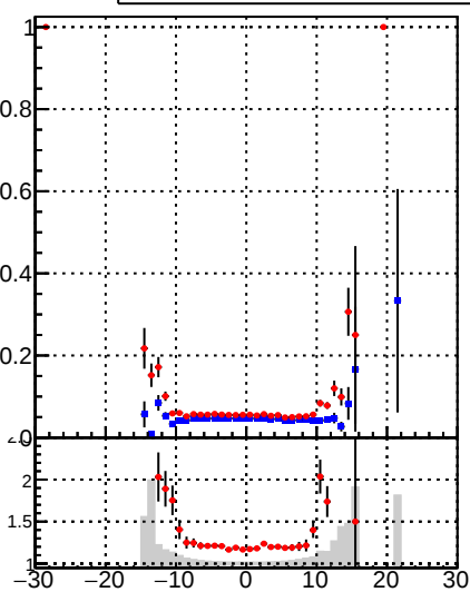
■ DQM_mkFit ● DQM_BDT_mkFit
