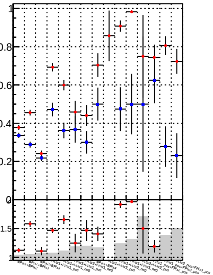
Fake rate vs. DQM mkFit DQM BDT mkFit
