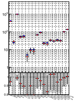
N of reco track vs. s DQM mkFit DQM BDT mkFit
