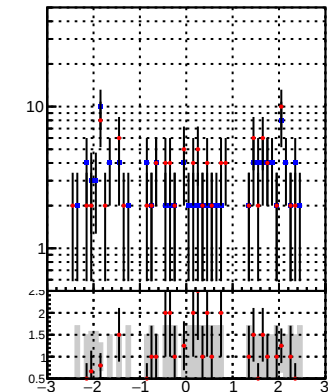
pT eta
