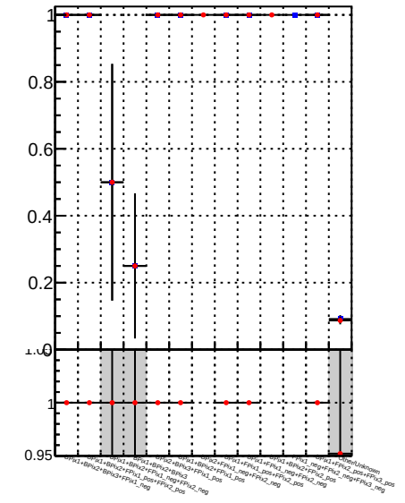
Fake rate vs. —●— DQM mkFit —●— DQM BDT mkFit
