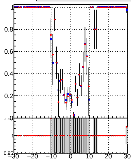
— DQM_mkFit — DQM_BDT_mkFit
