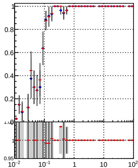
— DQM_mkFit — DQM_BDT_mkFit
