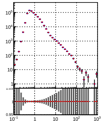
—●— DQM_mkFit —●— DQM_BDT_mkFit
