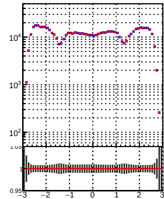
—●— DQM_mkFit —●— DQM_BDT_mkFit
