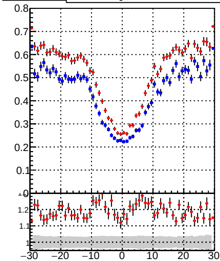
◆ DQM_mkFit ★ DQM_BDT_mkFit
