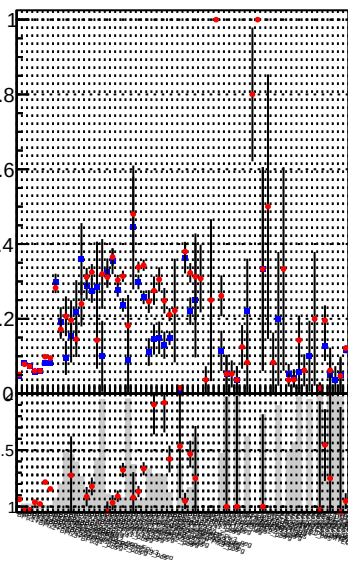
Fake rate vs. DQM mkFit DQM BDT mkFit
