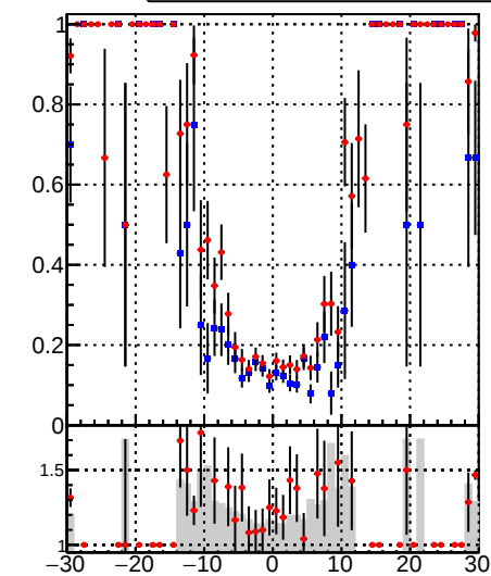
■ DQM_mkFit ● DQM_BDT_mkFit
