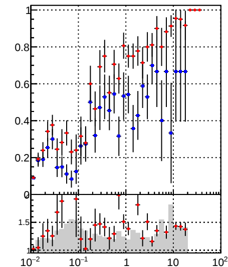
■ DQM_mkFit ● DQM_BDT_mkFit
