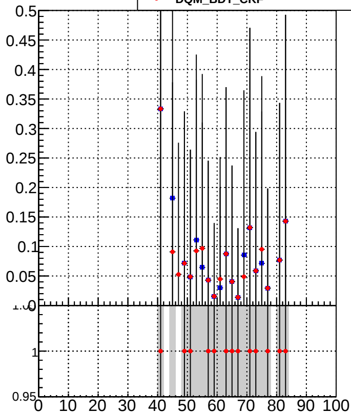
DQM_CKF DQM_BDT_CKF
