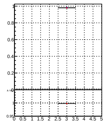
Fake rate vs hit DQM_CKF DQM_BDT_CKF
