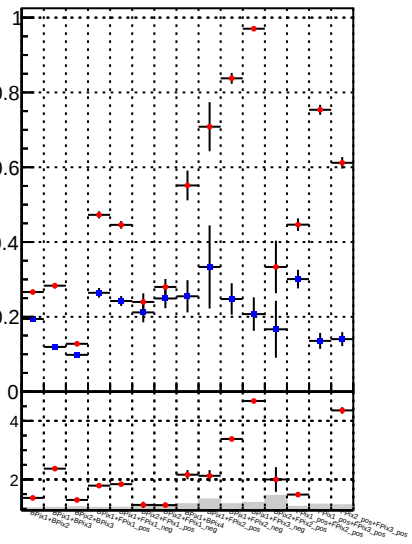
Fake rate vs. — DQM CKF — DQM BDT_CKF
