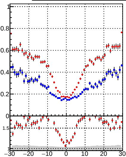
DQM_CKF DQM_BDT_CKF
