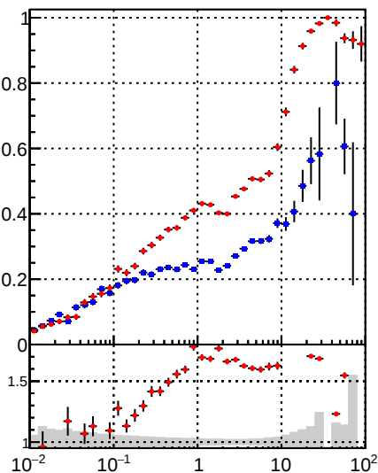
DQM_CKF DQM_BDT_CKF
